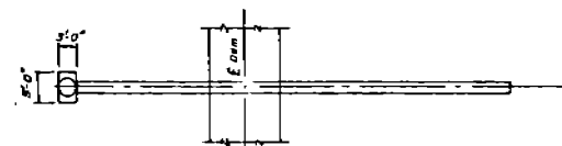
PLAN OUTLET CONDUIT AND RISER
